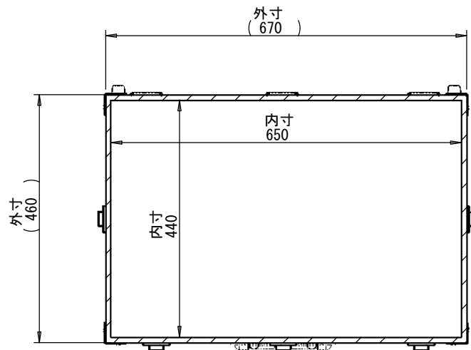
断面図 A-A
