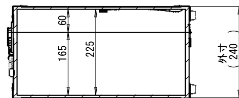
断面図 B-B
