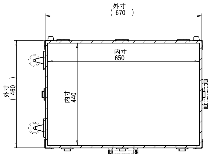
断面図 A-A
