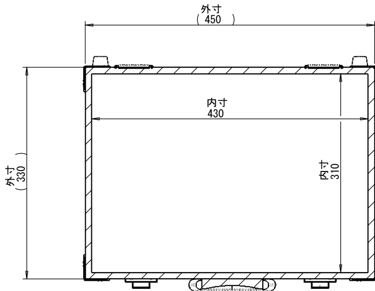
断面図 A-A スケール 1:6
