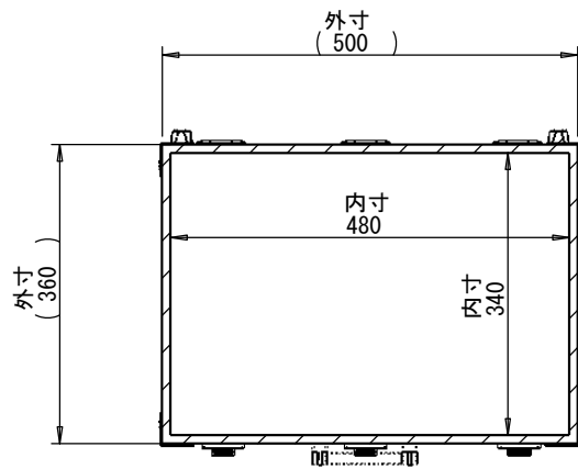
断面図 A-A
