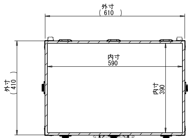
断面図 A-A
