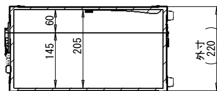
断面図 B-B
