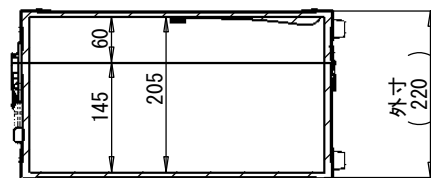
断面図 B-B
