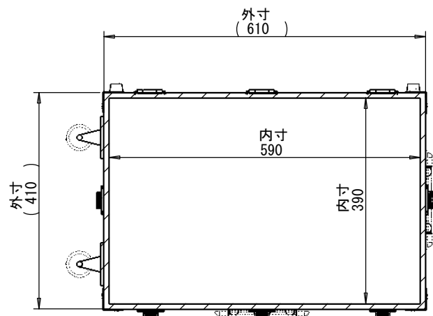
断面図 A-A
