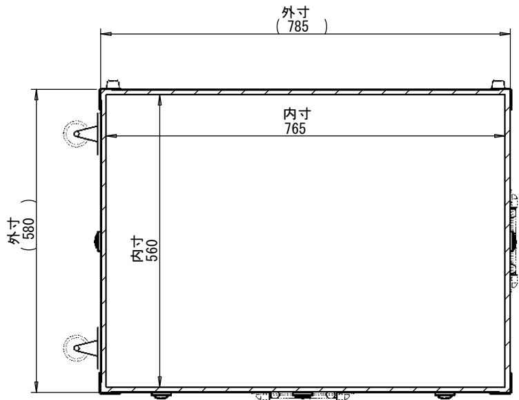
断面図 A-A
