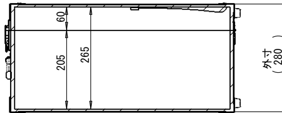
断面図 B-B
