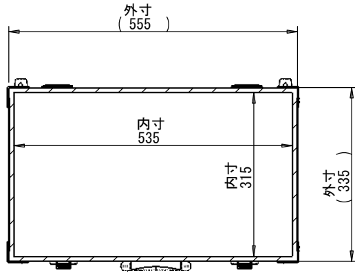
断面図 A-A
