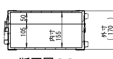
断面図 B-B
